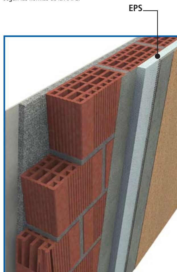
Placa Exterior Sistema EIFS
